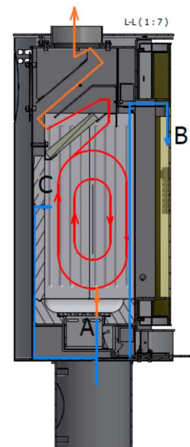
Lufts.2.2 Luftstrom – Beispiel ARCO F1
