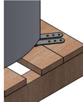
Abb. 1.2. Befestigen des Heizgeräts an der Palette
