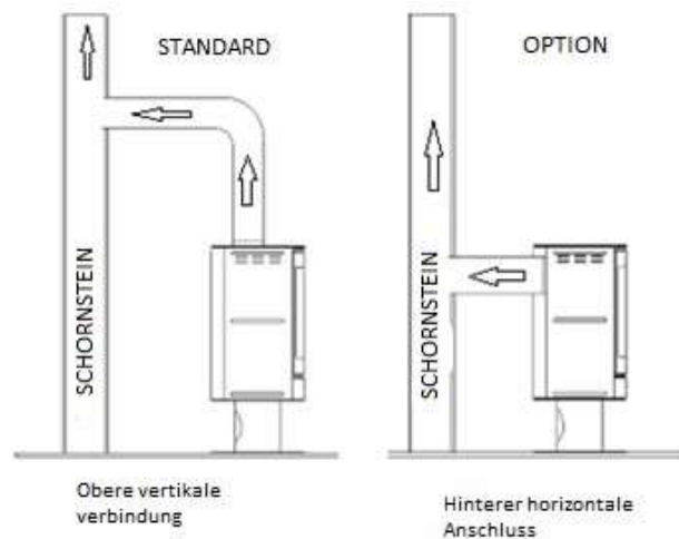
Abb. 3.5. Methoden zur Installation der Luftzufuhr und Abgasabfuhr
