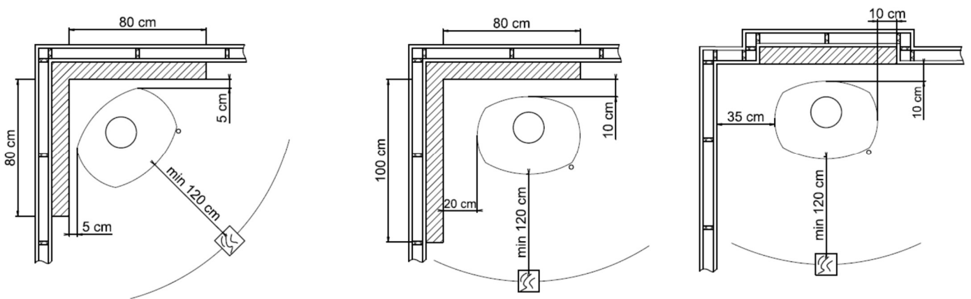
Abb. 3.3. Mindestabstand zu einer brennbaren Wand, geschützt durch eine Schutzwand
