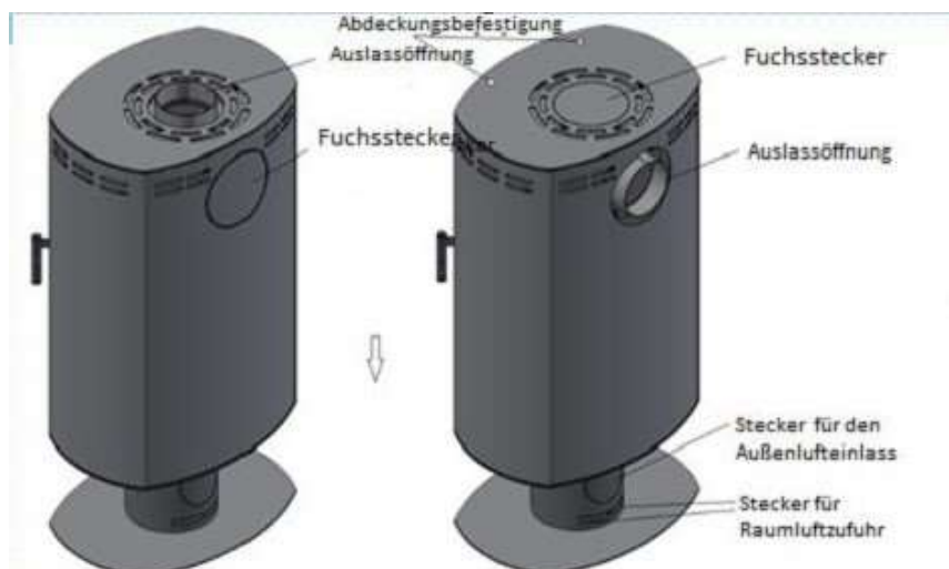
Abb. 3.6. Lage des Abgasaustritts Beispiel ARCO F1
