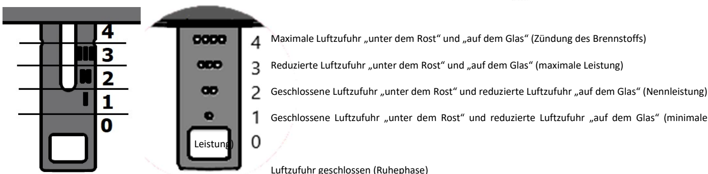
Abb. 4.1. Standort des Luftreglers
