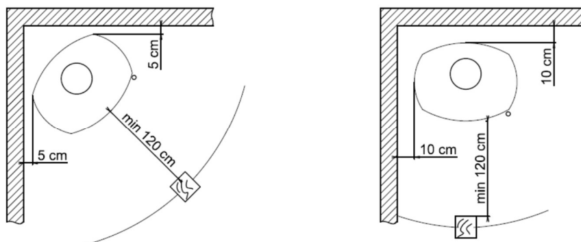
Abb. 3.4. Mindestabstand zu einer nicht brennbaren Wand
