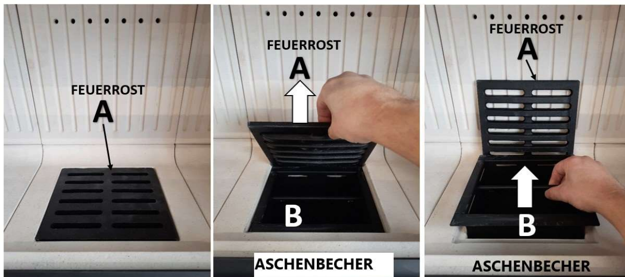
Abb. 4.3 Asche entleeren
